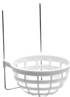
NIDO INTERNO cm 10 x 11 x 16h EAN: 8033844760474 Cod: AC400116 Art.039
